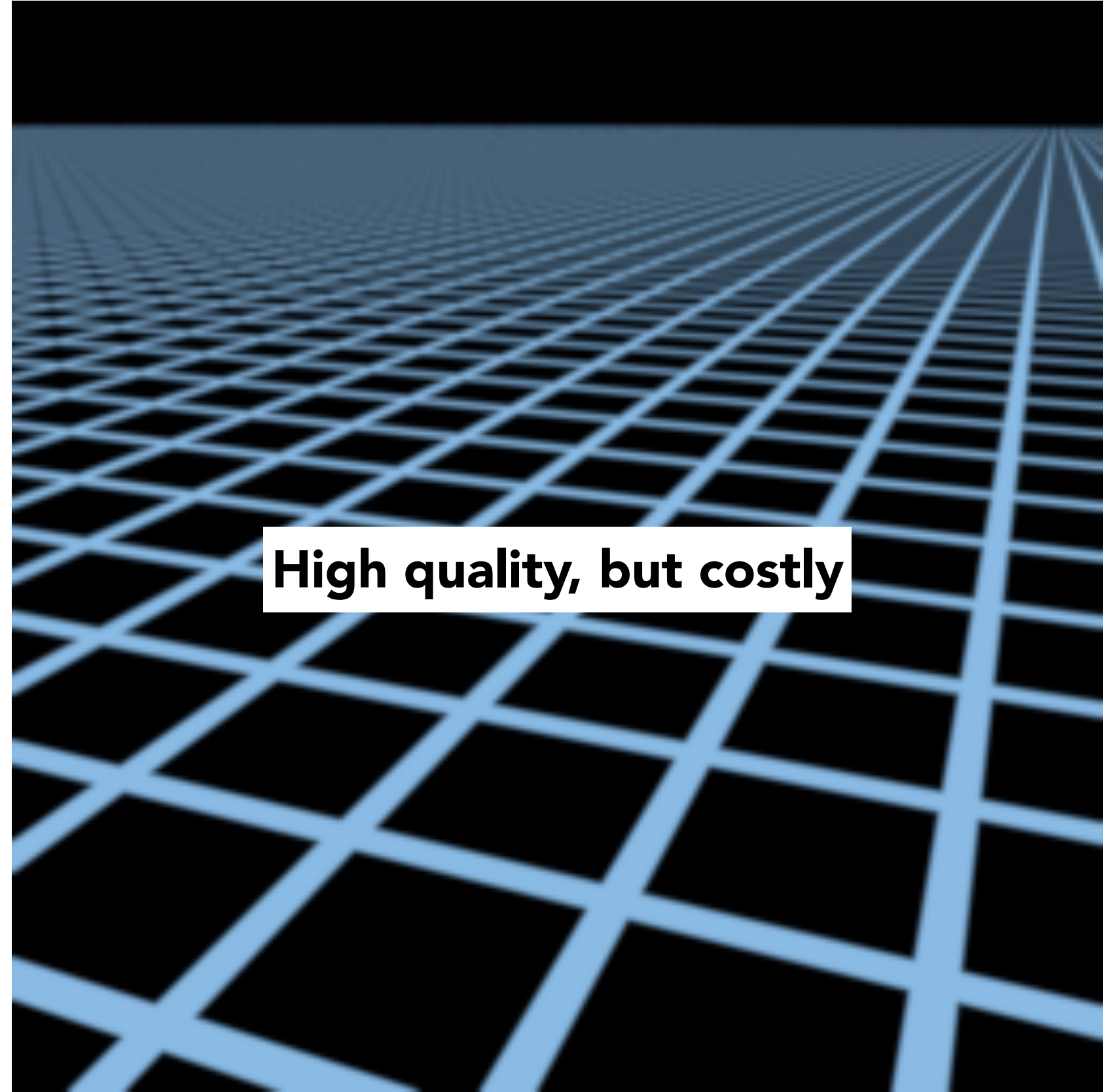
512x supersampling
